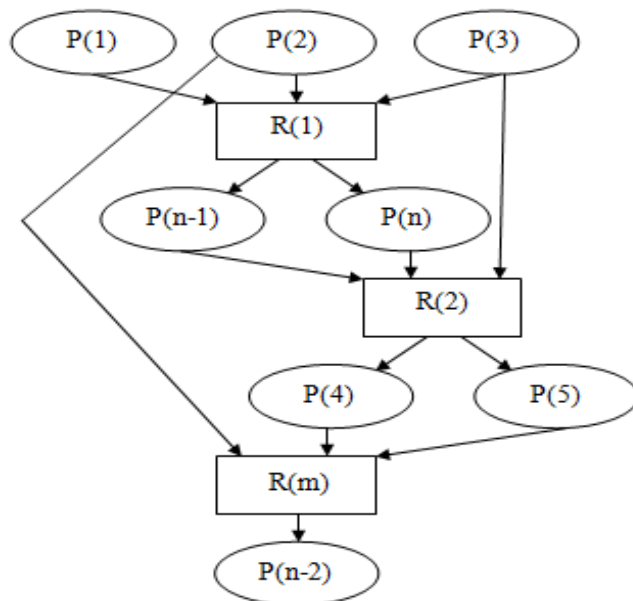
Рисунок 20 - Иллюстрация при помощи двудольного графа шага №7
