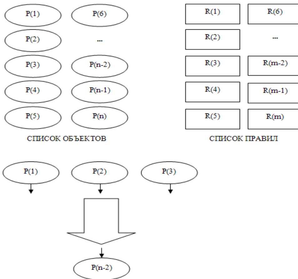
Рисунок 8 - Иллюстрация при помощи двудольного графа шага №1
