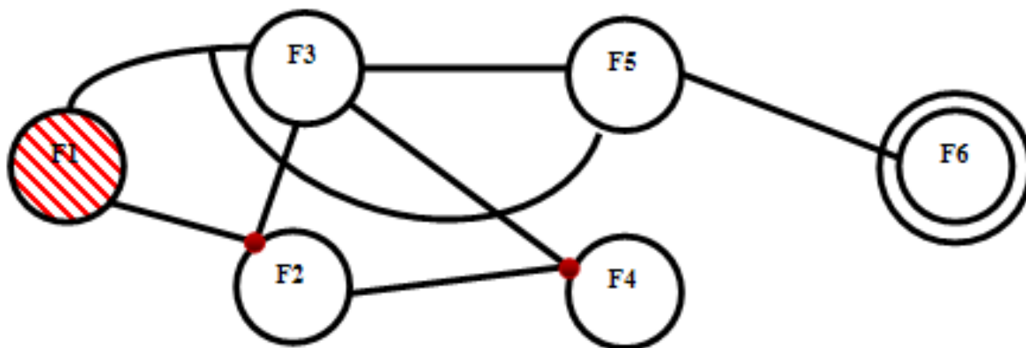
Рисунок 1 - Пример однодольного графа неориентированной "И-ИЛИ сети"
