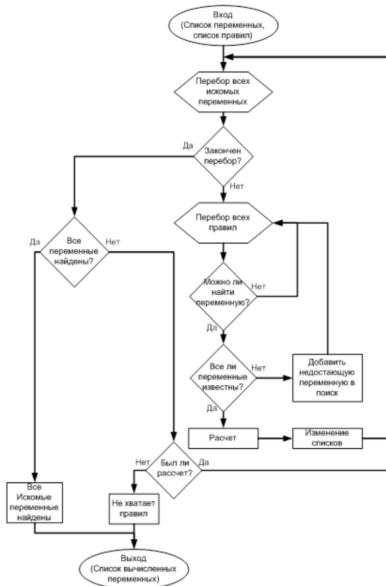
Рисунок 4 - Алгоритм миварной логико-вычислительной обработки для ПК УДАВ
