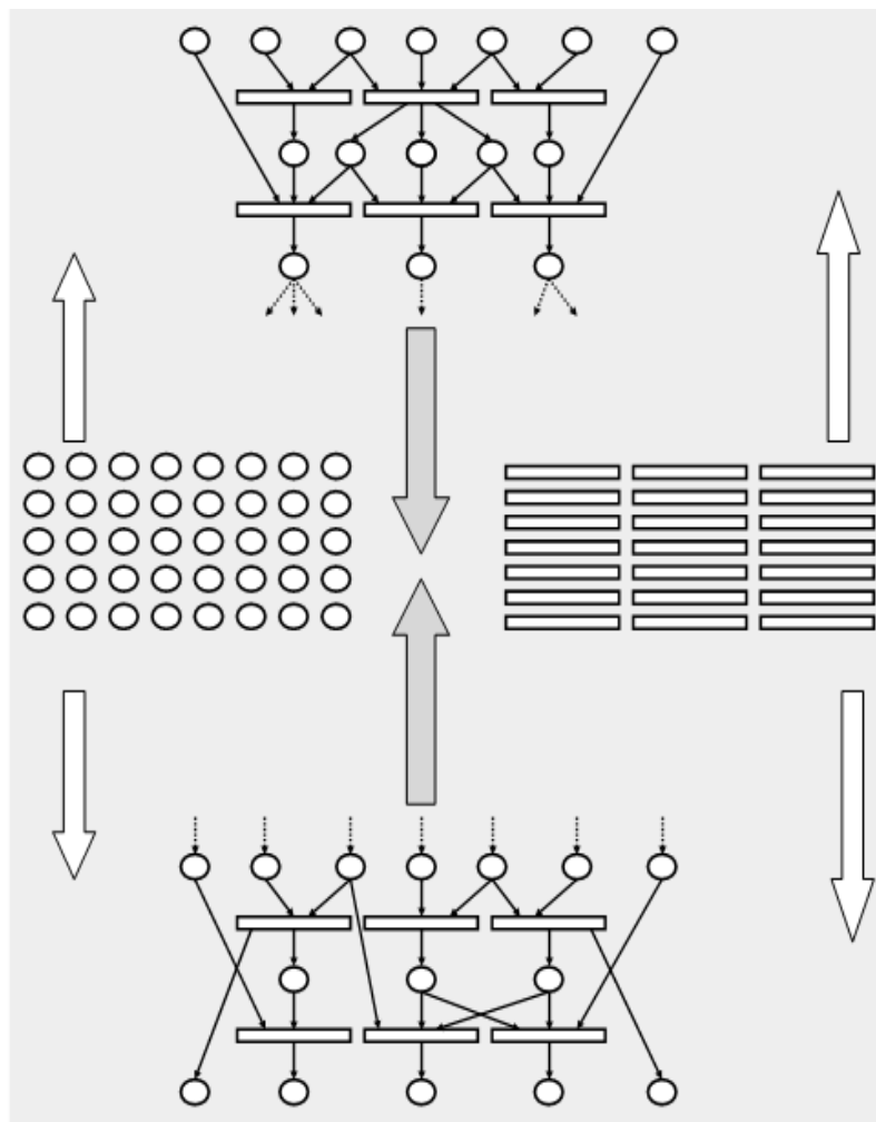
Рисунок 2 - Представление миварной сети в виде двудольного графа
