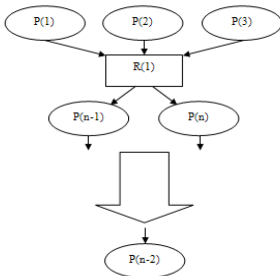
Рисунок 12 - Иллюстрация при помощи двудольного графа шага №3
