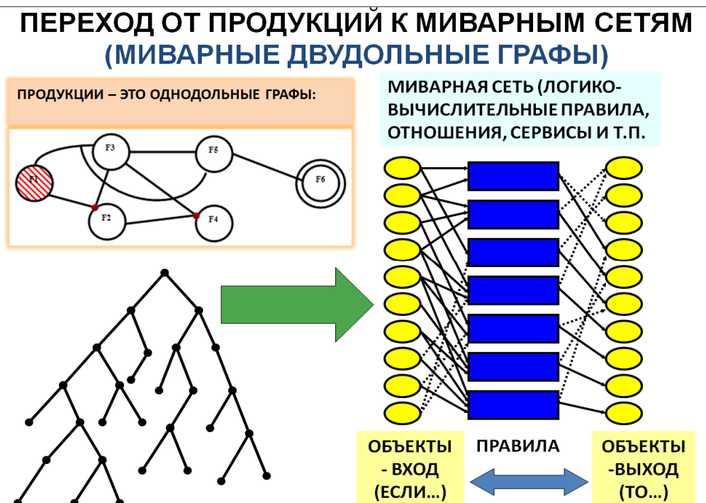
Рисунок 22 - Переход от продукций к миварным сетям
