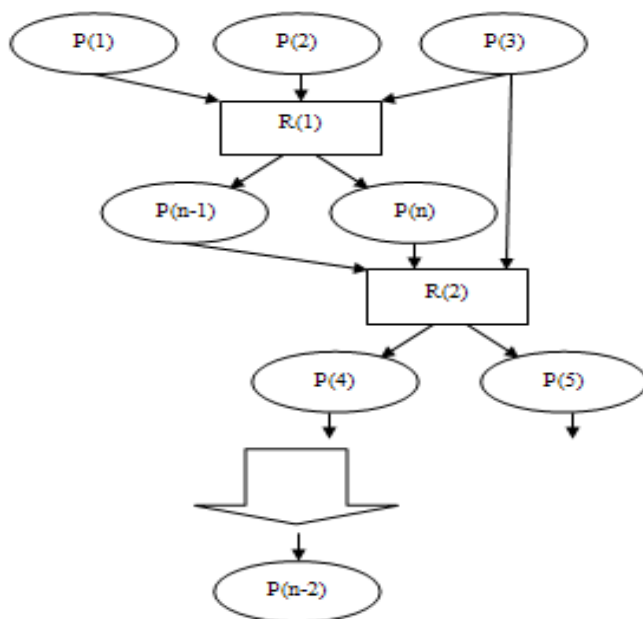
Рисунок 16 - Иллюстрация при помощи двудольного графа шага №5
