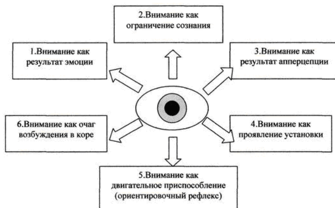
Рис. 1. Гипотезы внимания
