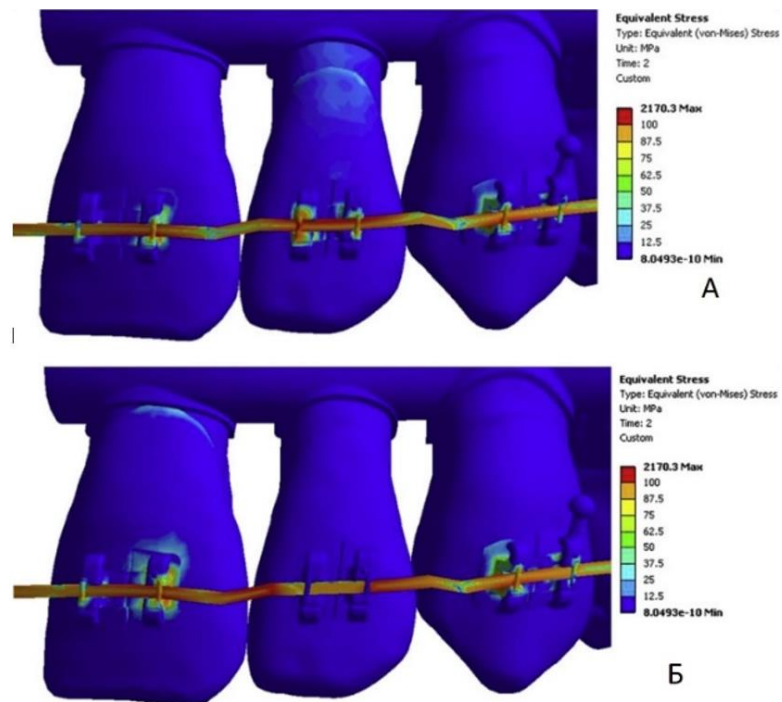
Рис. 16. Еквівалентна напруга за Мезісом на контакті дроту та брекетів: А – у моделі одношаровій, Б – у багатошаровій моделі
