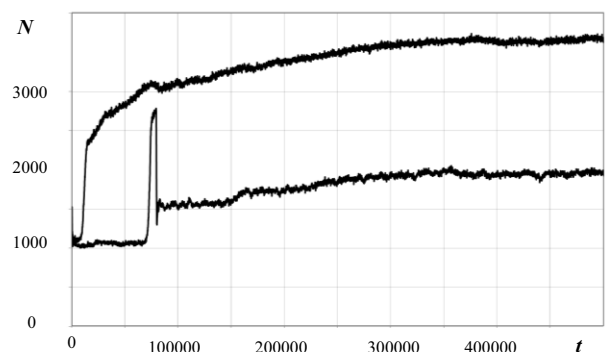
Рис. Зависимость численности популяции N от времени t в полной модели (нижняя кривая) и в случае «глобального пацифизма» (верхняя кривая).
