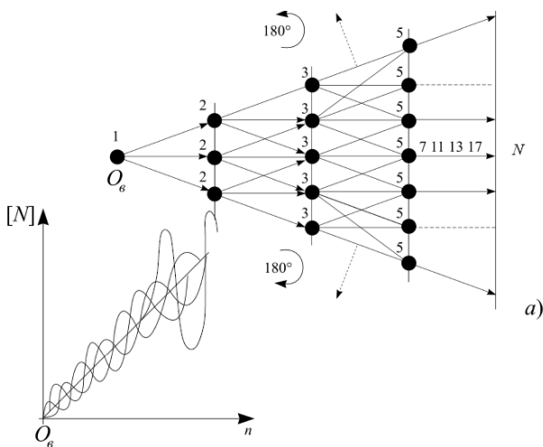
Рис. 4. Запись ФКВ на галактиках (верхний иерархический уровень) с последовательным расширением трехмерных матриц простых чисел (а) и волновое рассеяние матриц [N] (б) (O B – см. подпись к рис. 2)
