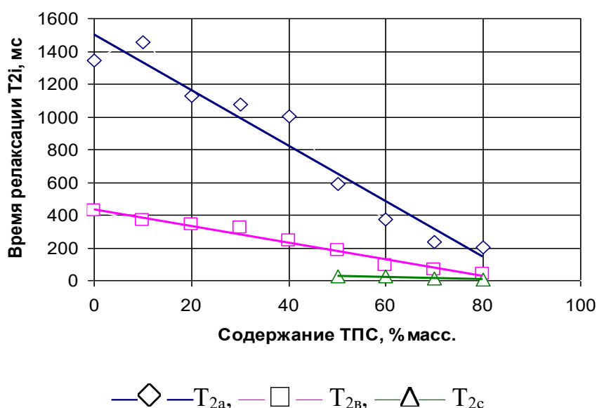
Рисунок 1 - Зависимость времен спин-спиновой релаксации T_{2i} от содержания ТПС в растворе ПВМ при 140 °С
