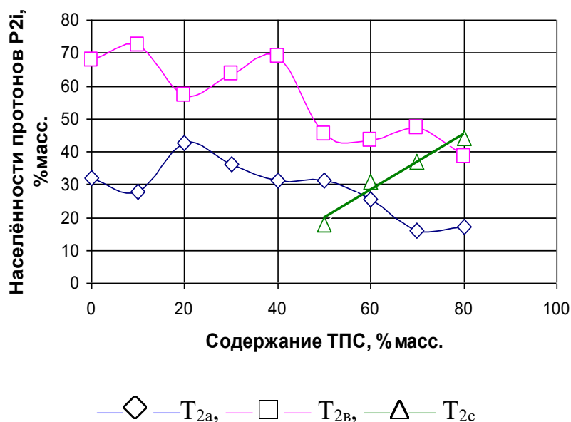
Рисунок 2 - Зависимость населённостей протонов фаз P_{2i} от содержания ТПС в растворе ПВМ при 140 °C
