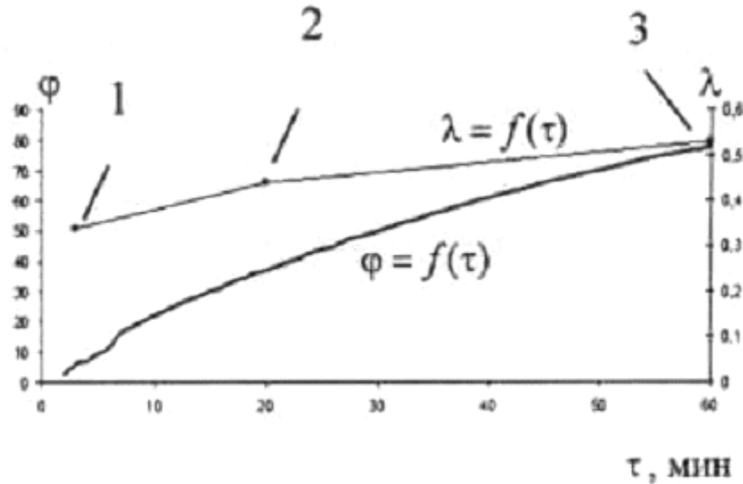
Рис. 4 Результаты исследований ТФХ сорбента на основе KO_2
