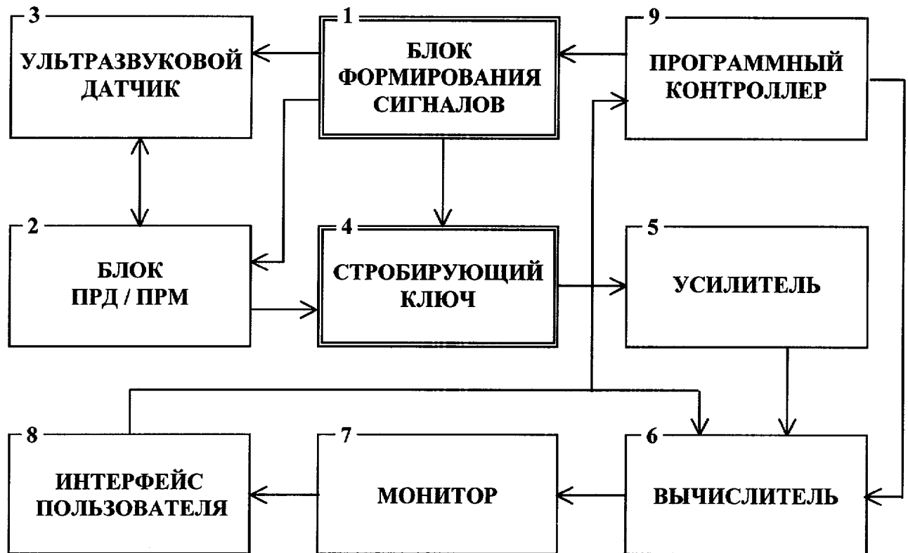
Рис. 2. Структурная схема акустического маммографа
