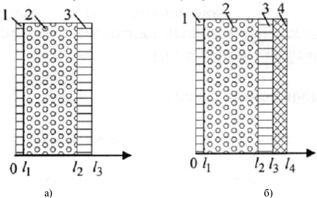
Рис. 3. Физическая модель ИА 1,3 – воздухопроницаемые оболочки; 2 – хемосорбент, 4 – защитная оболочка
