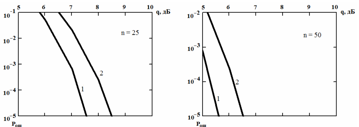
Рис. 4. Зависимости вероятности ошибки от отношения сигнал/шум (оптимальный алгоритм).
