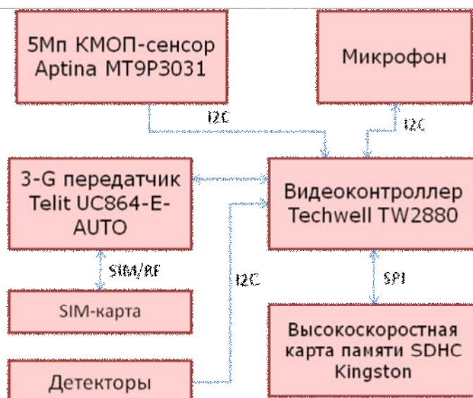
Рис. 1. Функциональная схема устройства
