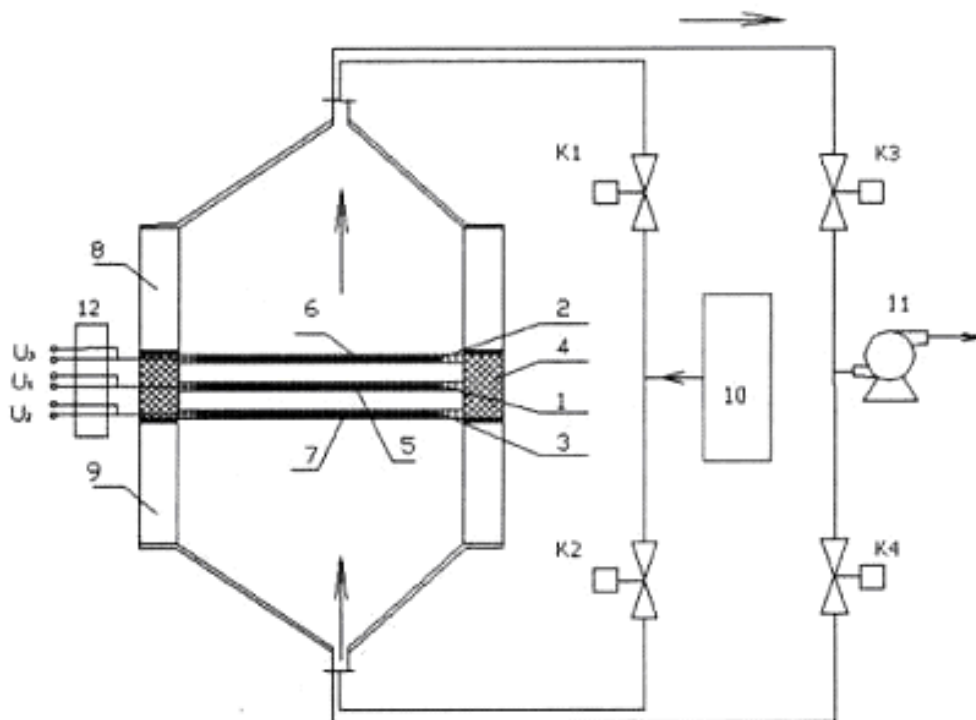
Рис.1. Схема установки для подготовки пробы
