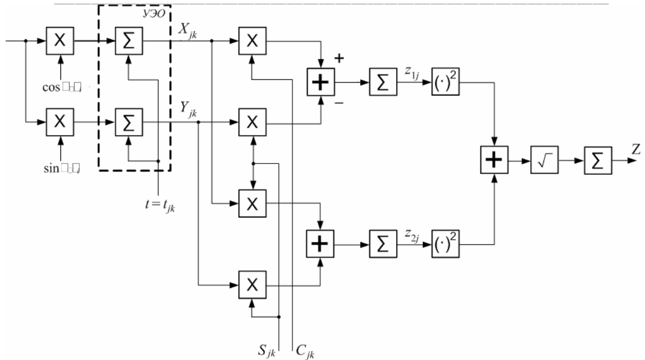
Рис. 2. Структура канала поиска квазиоптимального приёмника МЧМ-ШПС
