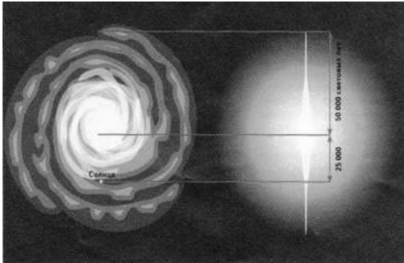
Рис.3.Наша Галактика Наша Галактика относится к спиральным. А в этих самых спиральных ветвях смежных галактик обычно происходят явно бурные процессы, которые активно порождают мощное излучение. ( Наше Солнце находится в относительно спокойном месте смежной Галактики и явно не испытывает интенсивного катастрофического
