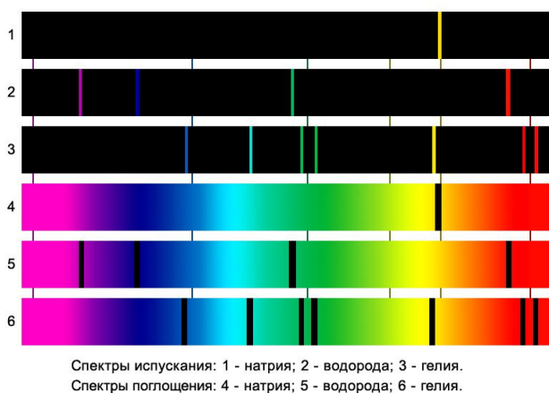
Рис.2. Спектры излучения и поглощения атомов: натрия, водорода, гелия.
