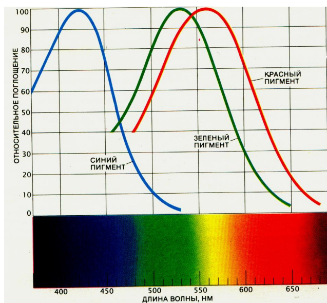
Рис.1. Спектр света и его относительное поглощение чувствительными пигментами сетчатки глаза человека [«В мире науки», №4, 1989г].
