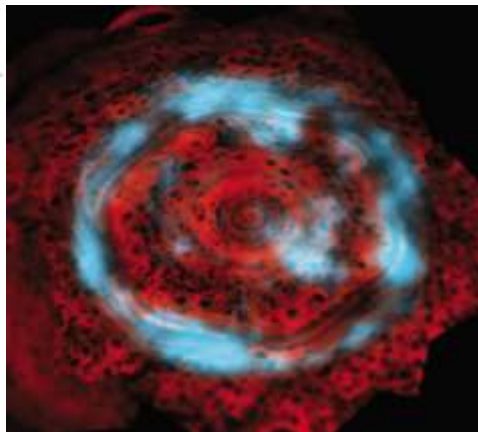
Рис.9. Северное сияние на Сатурне, полученное аппаратом Кассини в 2007году. Чётко виден шестигранник над полюсом планеты и светящийся овал в его границе.
