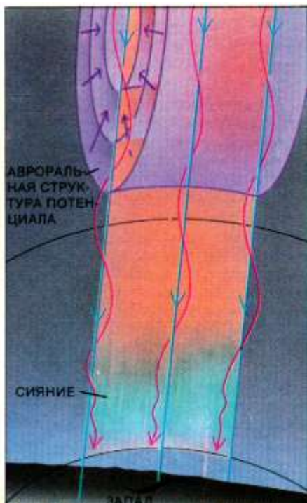
Рис.13. Плазменный механизм струйного потока электронов из магнитосферы Земли. Это зародыш мощного циклона, засасывающего солнечный ветер межпланетного магнитного поля.[9].
