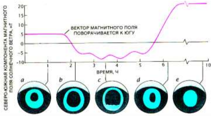
Рис.10. Фазы изменения овала полярного сияния над северным полюсом планеты, где расположен ЮЖНЫЙ магнитный полюс. [9].
