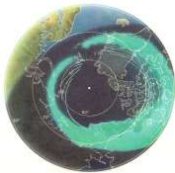
Рис.11. Изображение полярного овала, смещённого относительно географического полюса в сторону магнитного полюса Земли.[9].
