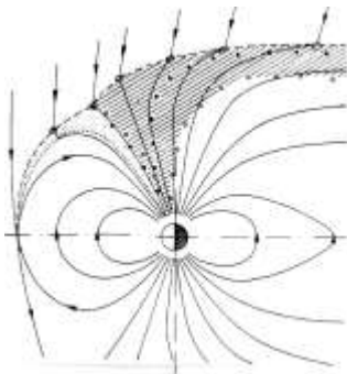
Рис.8. Представлена схема плазменной мантии и входного слоя в модели активной магнитосферы, открытой для работы с солнечным ветром. На рисунке заштрихована область дневной стороны магнитосферы, постепенно расширяющейся как опахало для втягивания частиц солнечного ветра.
