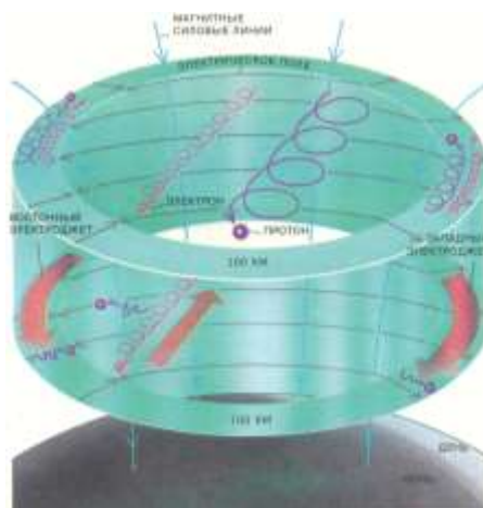
Рис.12. Схема энергии над полюсом планеты
