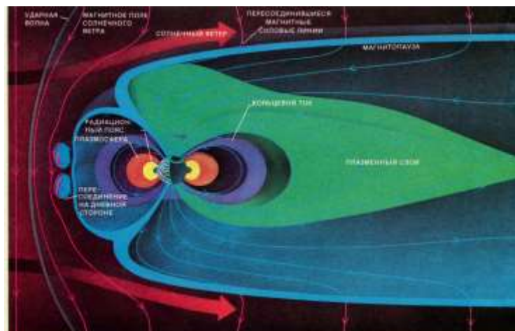
Рис.5. Схема чувствительной оболочки планеты – магнитосферы, радиационного пояса, ионосферы. [9].
