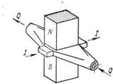
Рис. 7. Кондукционный электромагнитный насос по перекачке расплавленных металлов [6].
