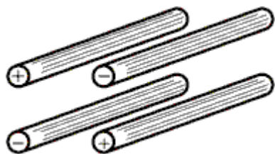
Рис. 2. Взаимное расположение стержней в квадрупольном конденсаторе мазера.
