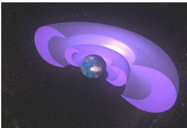
Рис.11 Радиационный пояс Земли. Он же плазменный объёмный резонатор единой квантовой системы генератора/усилителя – планеты Земля.
