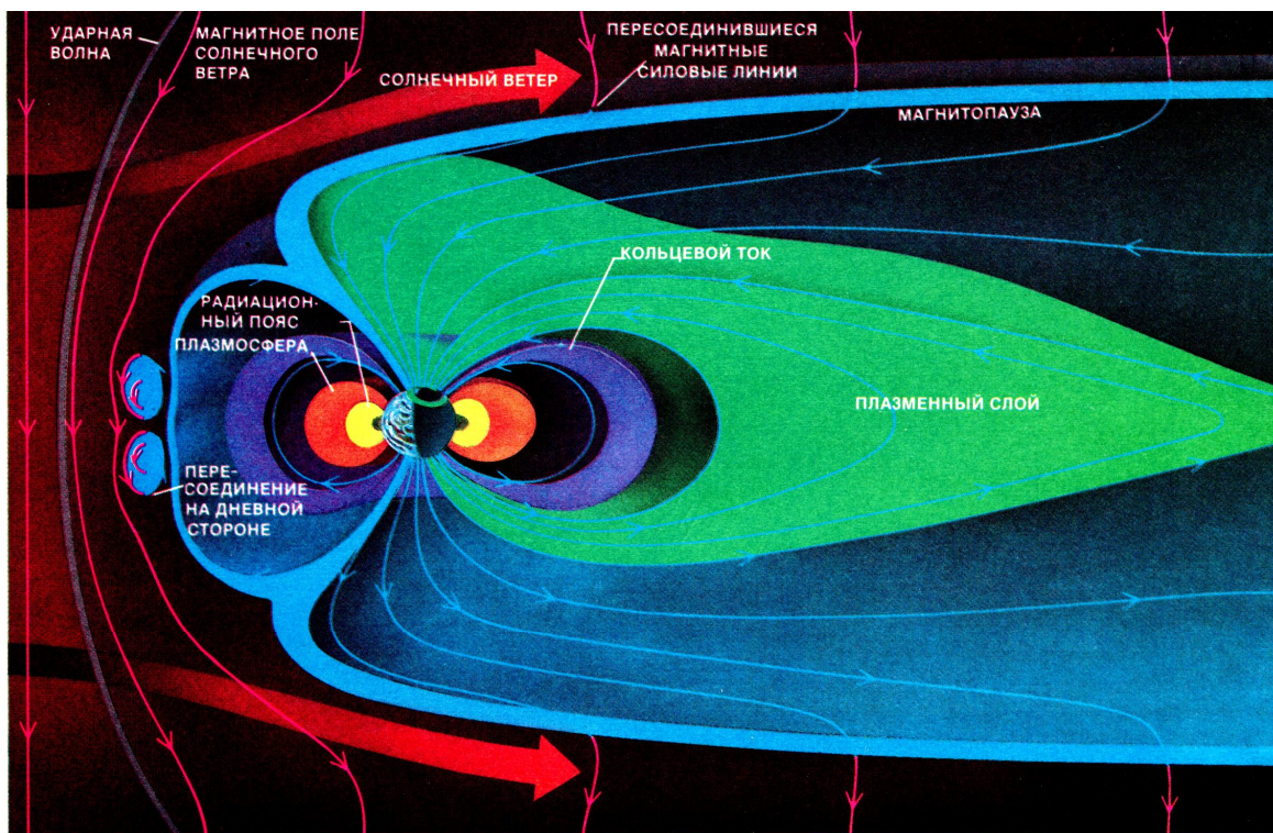
Рис.9. Магнитосфера Земли 14 – невидимый плазменный механизм Солнечно-Земных связей.
