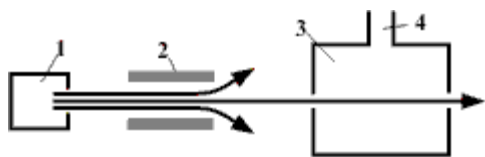
Рис. 1. Схема работы мазера на аммиаке. Прибор работает в условиях глубокого вакуума. 1 – источник возбужденных молекул аммиака. 2 – электрический селектор молекул по степени возбуждения. 3- объемный резонатор. 4 – вывод излучений из резонатора.
