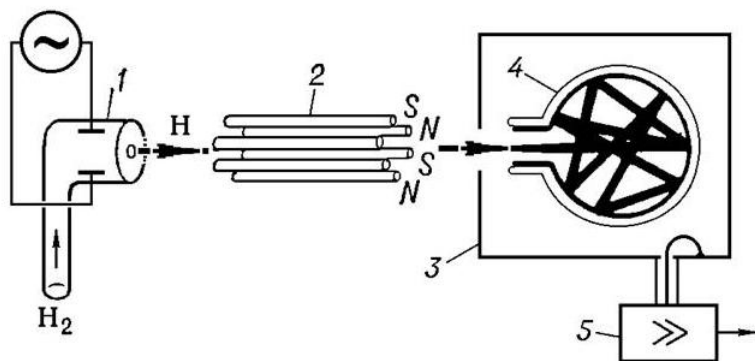
Рис. 3. Схема работы мазера на водороде. Показано, что в кварцевой колбе собираются атомы водорода, отдавшие своё возбуждение
