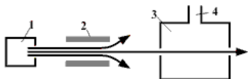
Рис. 1. Схема работы мазера на аммиаке. Прибор работает в условиях глубокого вакуума. 1 – источник возбужденных молекул аммиака. 2 – электрический селектор молекул по степени возбуждения. 3 - объёмный резонатор. 4 – вывод излучений из резонатора. Не показан путь возвращения молекул из области резонатора в источник возбуждения. В реальных условиях такой путь обозначен кругооборотом углерода между атмосферой и корой планеты.
