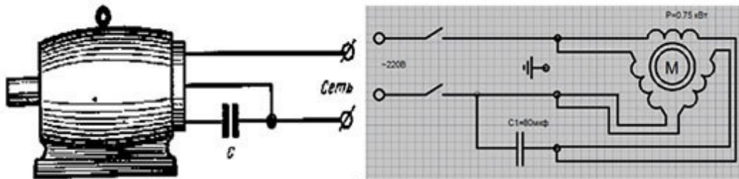
Схема подключения
