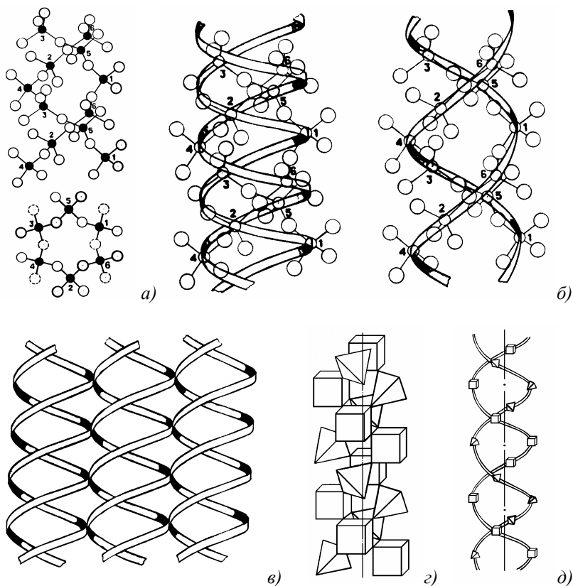
Рис. 18. Двойные спирали, топологически адекватные спиральям ДНК, в структурах неорганических веществ: проекция атомной структуры левого кварца (а); спиральная структура левого кварца (б); спиральное представление структуры кварца (в); фрагмент структуры упорядоченной шпинели (сорасположение тетраэдров и гексаэдров) (г); фрагмент структуры упорядоченной шпинели: двойная спираль из тетраэдров и гексаэдров (д) (по В. М. Таланову 119 ).
