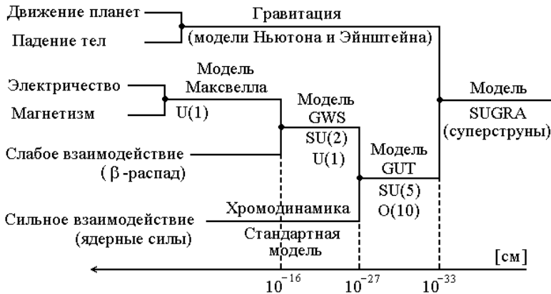
Рис. 9. Объединительная модель фундаментальных взаимодействий — на нижней оси указаны величины дальности действия в моделях (по Г. В. Клапдор-Клайнротхаусу и К. Цюберу 103 )
