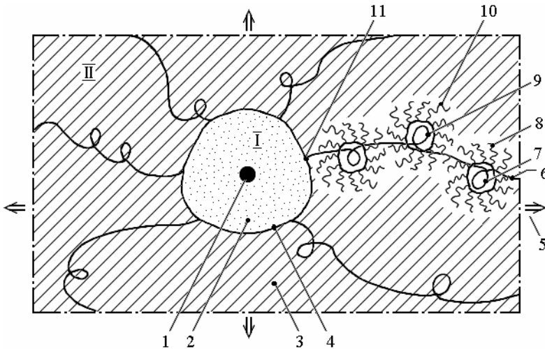
Рис. 15. К структурированию Вселенной: 1 — начальная сингулярность с бесконечно ( 1/0 = \infty ) большой плотностью; 2 — радиационно-доминантная фаза Вселенной (I); 3 — вещественно-доминантная фаза Вселенной (II); 4 — замкнутая физическая струна — фазовый переход I \rightarrow II ; 5 — расширение современной Вселенной; 6 — незамкнутая струна; 7 — D -петля струны 6; 8 — галактика с D -киральностью; 9 — L -петля струны 6; 10 — галактика с L -киральностью; 11 — триплет струн
