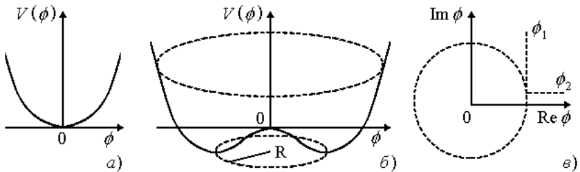
Рис. 10. К иллюстрации потенциала Хиггса: сохранение симметрии при невырожденном вакууме (а); вырождение вакуума (б); вид потенциала в плане комплексной плоскости (в) (по Г. В. Клапдор-Клайнгротхаусу и К. Цюберу 103 )
