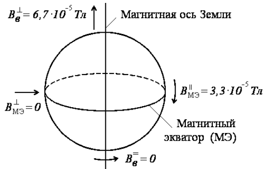
Рис. 19. Характеристики геомагнитного поля Земли ( B_g^{\perp} — максимальное значение индукции вертикальной составляющей магнитного поля на магнитных полюсах; B_g^{\parallel} — минимальное (нулевое) значение индукции горизонтальной составляющей магнитного поля на магнитных полюсах; B_{MЭ}^{\parallel} — максимальное значение индукции горизонтальной составляющей магнитного поля на МЭ; B_{MЭ}^{\perp} — минимальное (нулевое) значение вертикальной составляющей магнитного поля на МЭ).
